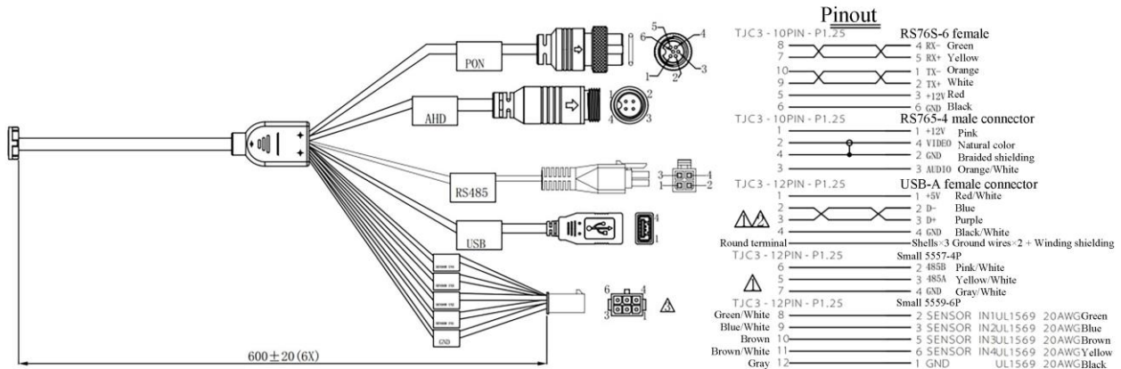
P3 V3.0-PON
